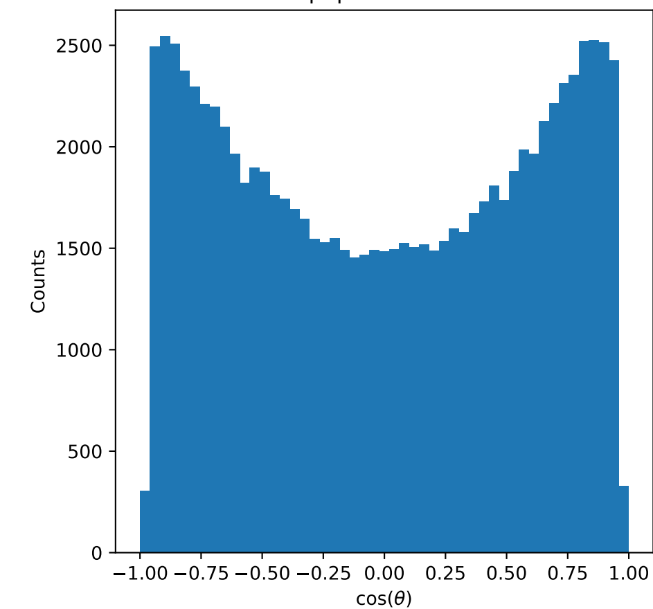
\mu^+\mu^- channel
