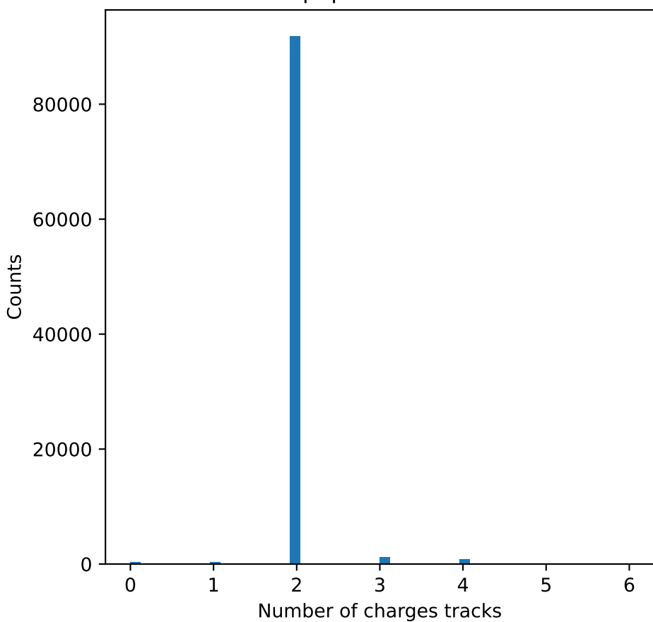
\mu^+\mu^- channel
